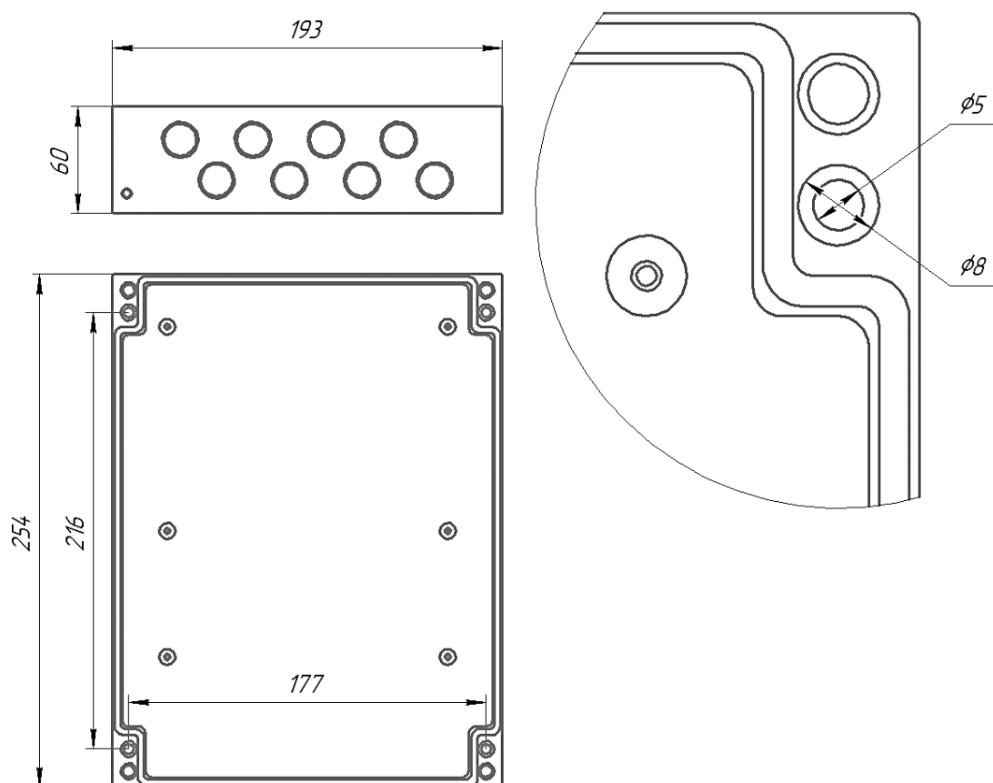
Рисунок 5: Габаритные и монтажные размеры контроллера
