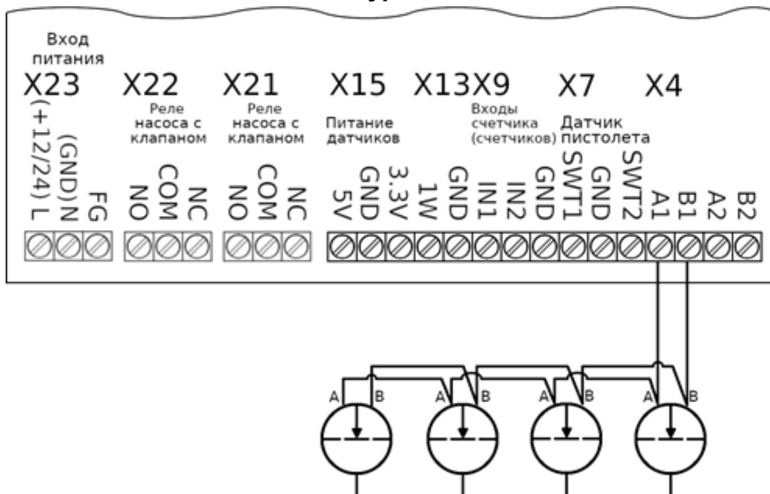
Рисунок 12: Схема подключения датчиков уровня
