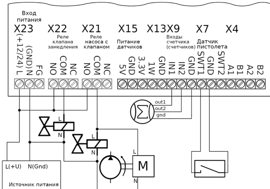
Рисунок 7: Схема подключения устройств в однопостовом режиме
