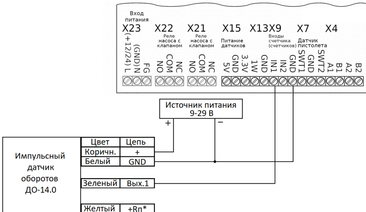
Рисунок 14: Схема подключения датчика оборотов ДО-14.0
