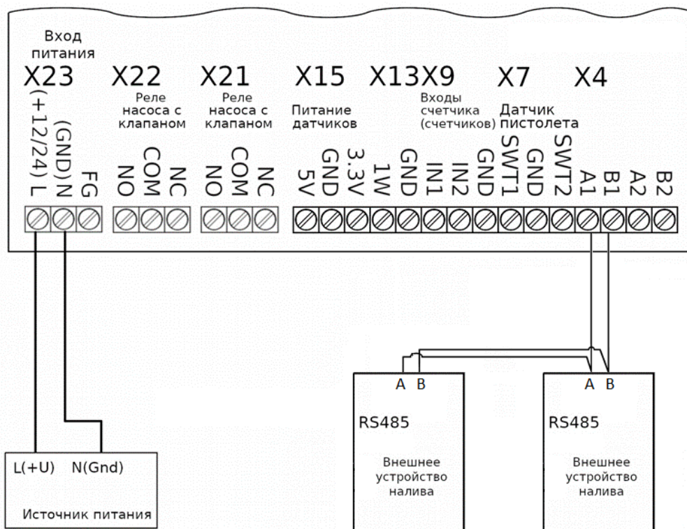
Рисунок 10: Схема подключения внешних устройств выдачи в двухканальном режиме
