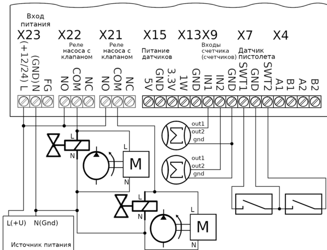
Рисунок 8: Схема подключения устройств в двухпостовом режиме
