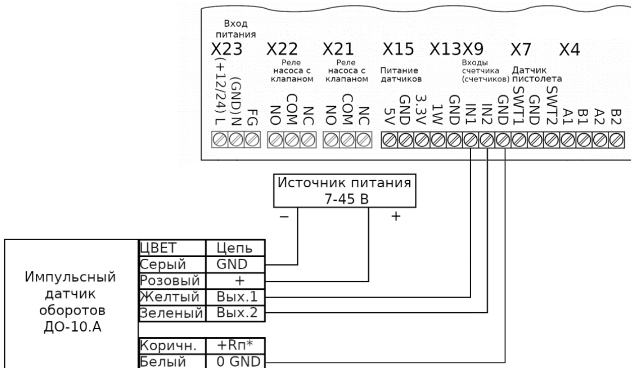
Рисунок 13: Схема подключения датчика оборотов ДО-10.А
