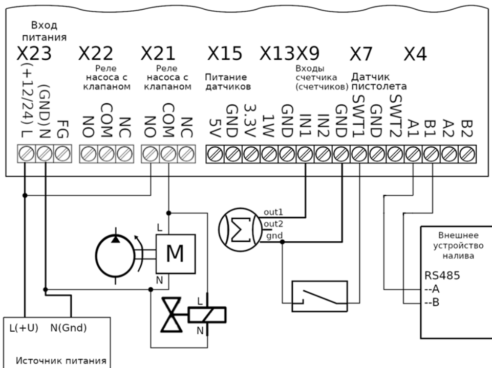
Рисунок 11: Схема подключения двухпостовая комбинированная.
