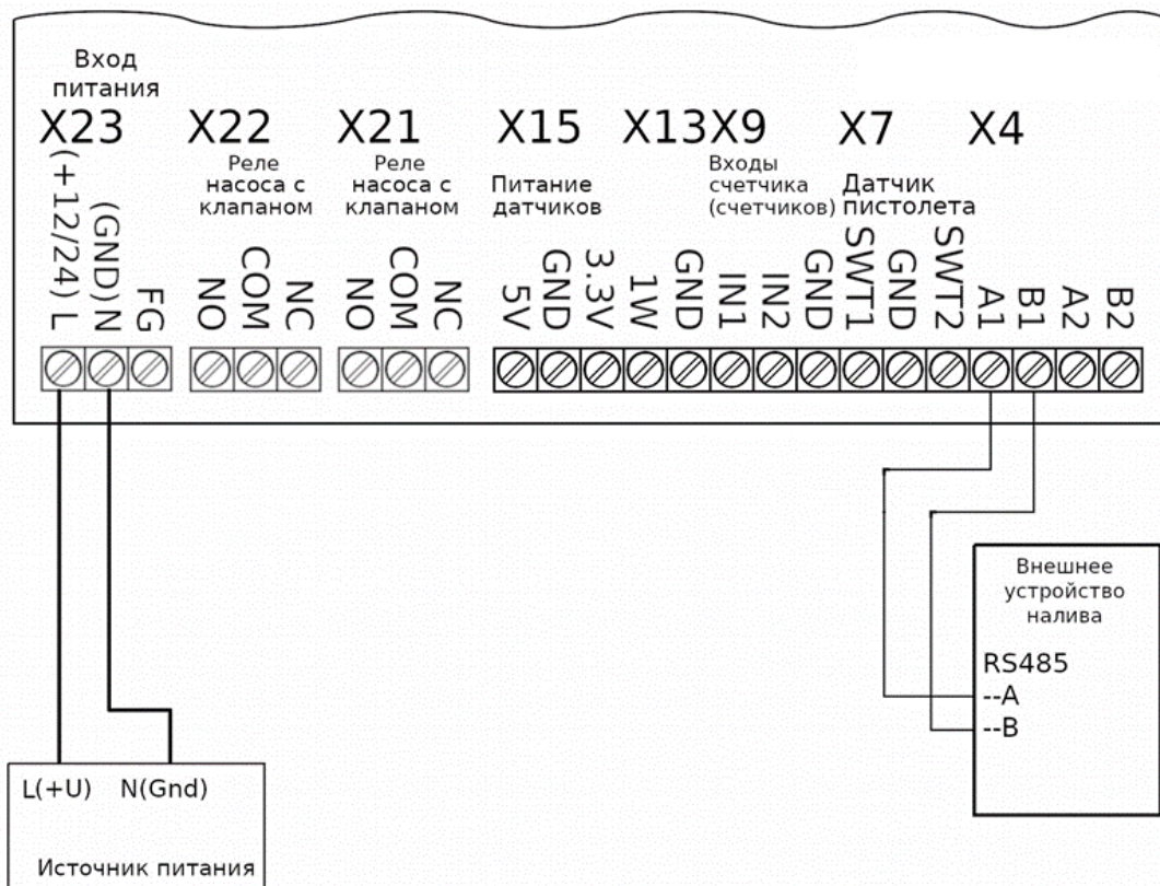
Рисунок 9: Схема подключения внешнего устройства выдачи в однопостовом режиме
